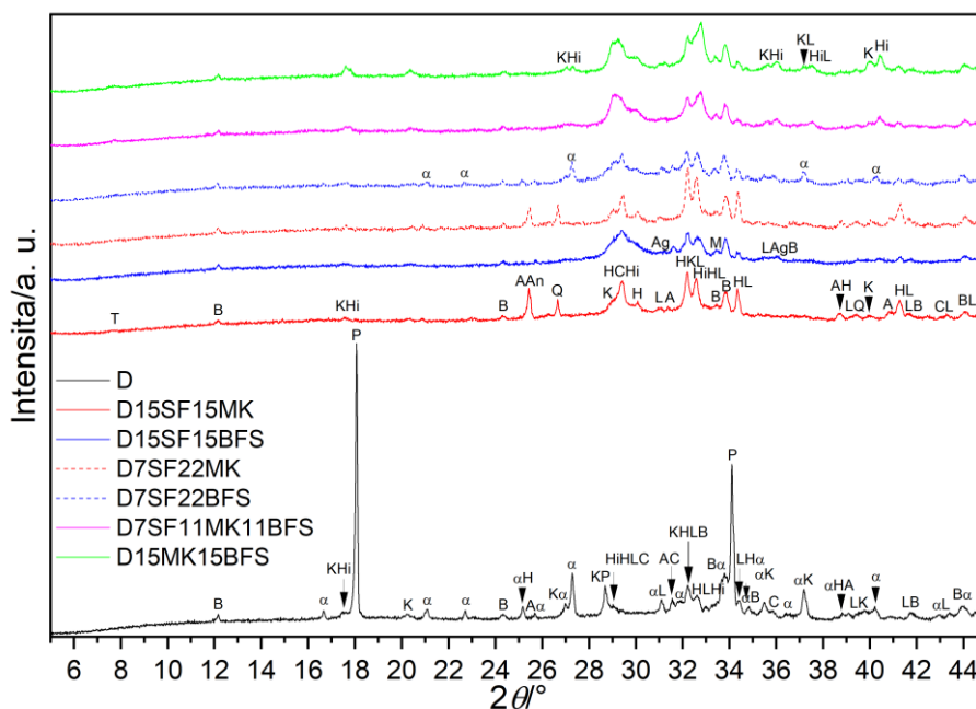
Obr. Záznamy röntgenovej difrakčnej analýzy študovaných cementových kompozitov.
